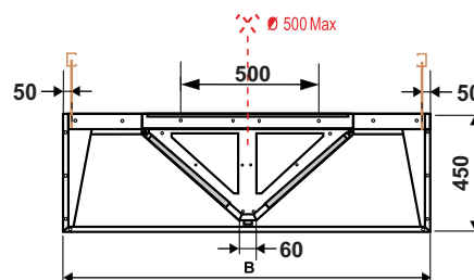
Hotte HILOT HC/V
